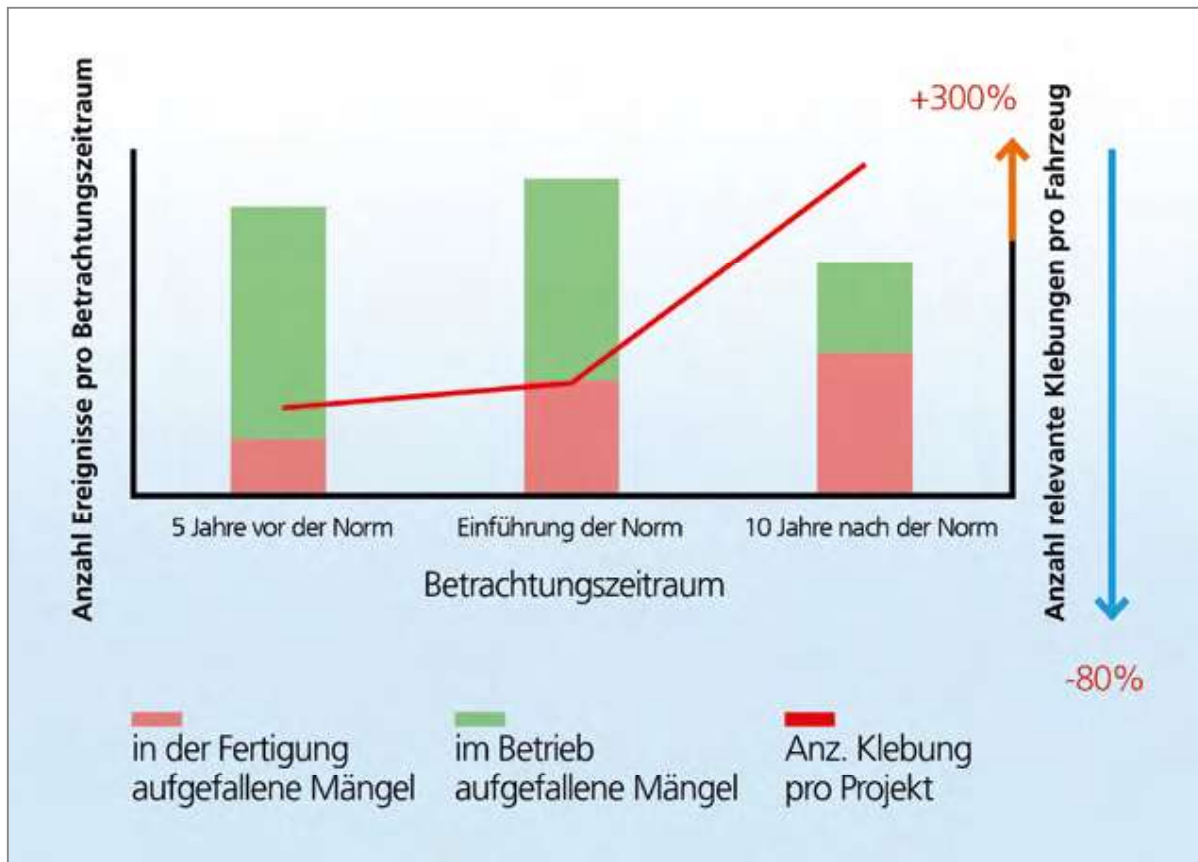
Bild 3: Langzeitstudie DIN 6701 (Bild: Fraunhofer IFAM | Bremen)
